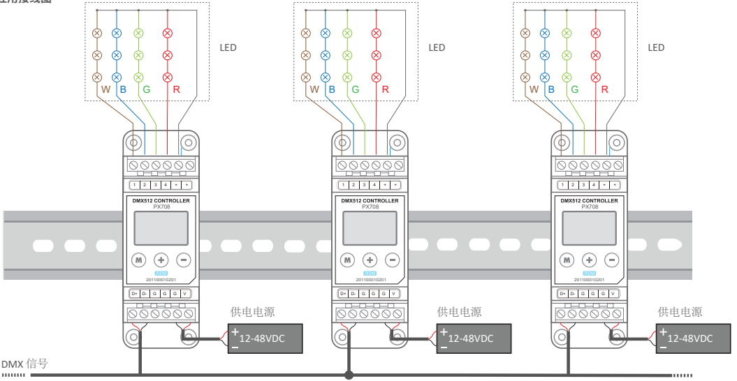
应用接线图
